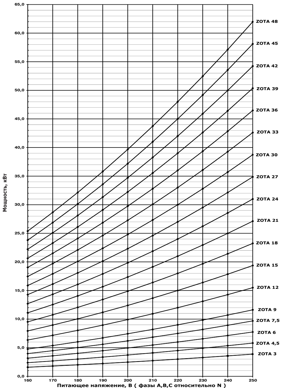
Рис. 11 График изменения мощности электроводонагревателя в зависимости от питающего напряжения
